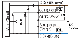
KP45 □ - 011 - □ 2 NPN + Analog Output(4~20mA)
